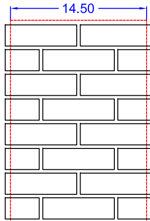
ELEVATION
